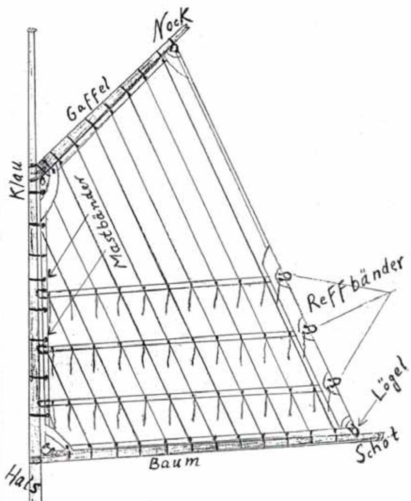
8.) Großsegel des früheren Norderneyer Lustfahrbootes „Arion“
