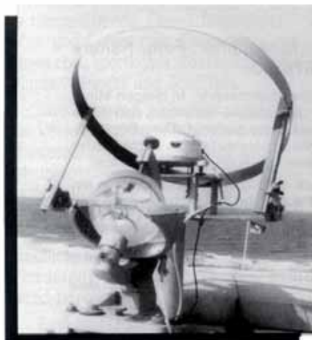
Meßinstrument für die Sonnenscheindauer
