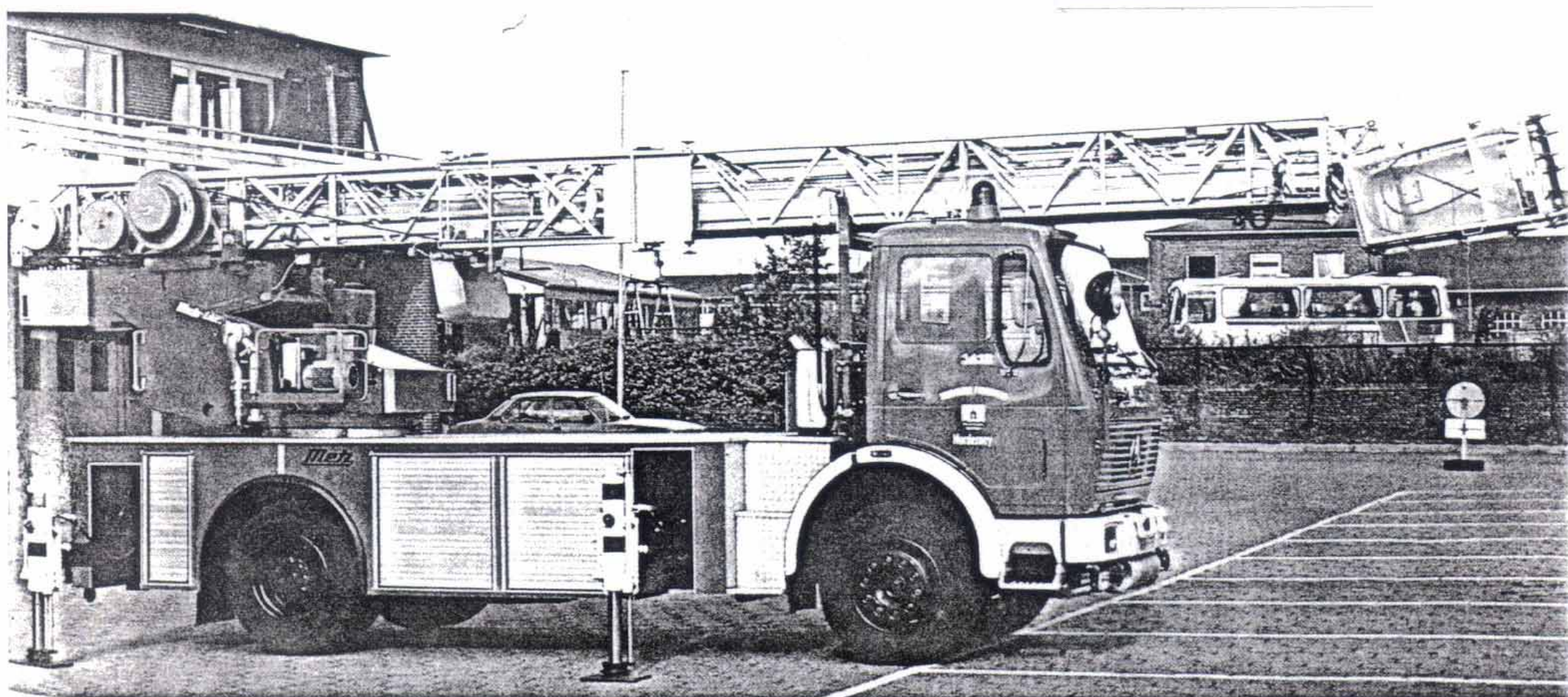
Drehleiter DLK 23-12, Aufbau Metz, Baujahr 1978.
