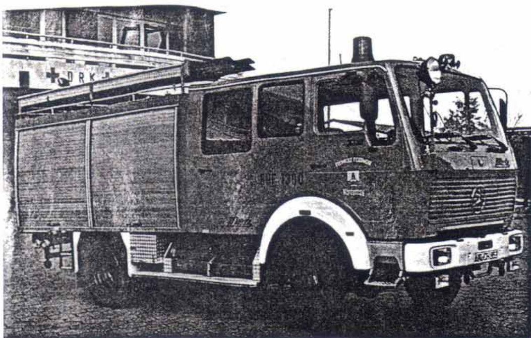
Das TLF 16, Mercedes 1019, Aufbau Metz, Baujahr 1979.
