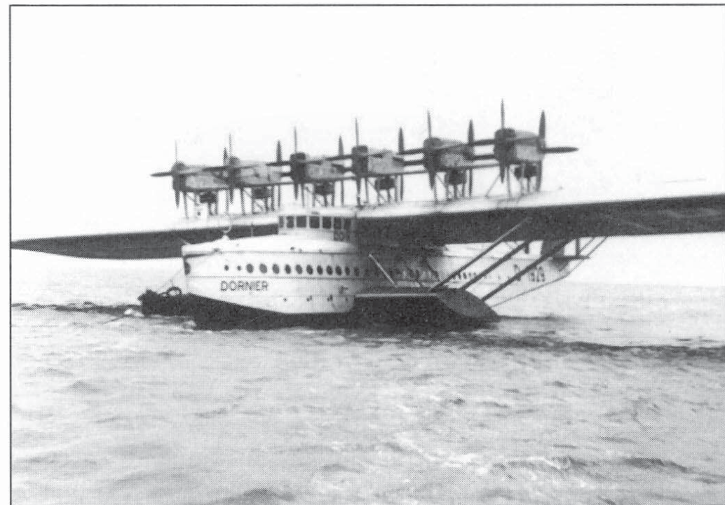
Abb. 4: Flugschiff DO-X ankert vor der Flugstation.
